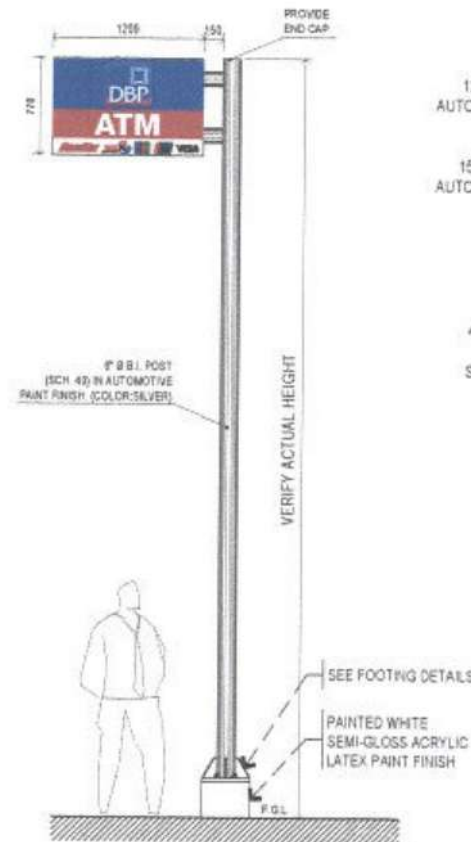
ELEVATION
