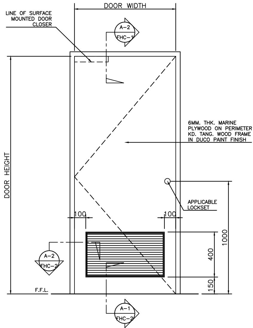
ELEVATION
