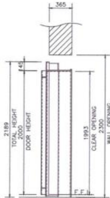
A-2 VDD-1 SECTION SCALE 1:30 M.
